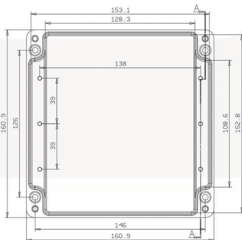
Gövde / Housing / بدنه
