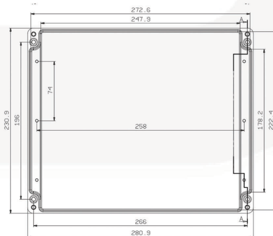
Gövde / Housing / بدنه
